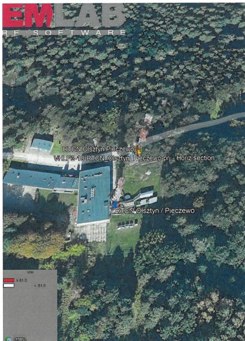
Rys. 2. Rzut poziomy rozkładu pola elektromagnetycznego anteny nowo projektowanej linii radiowej w otoczeniu RTCN Olsztyn / Pieczewo przewidzianej do zainstalowania na wysokości 215 m nad poziomem terenu.
