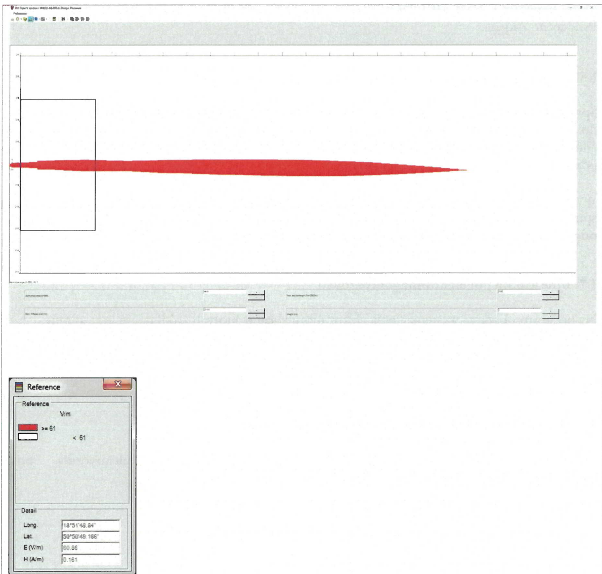
Rys.1. Rozkład poziomów pola elektromagnetycznego w otoczeniu nowo projektowanej linii radiowej w przekroju pionowym.
